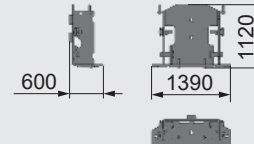
Gegengewichtskonsolle 0,5 t Support bracket for counterweight 0.5 t
