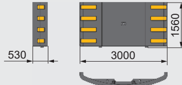
Gegengewicht 4,1 t Counterweight 4.1 t
